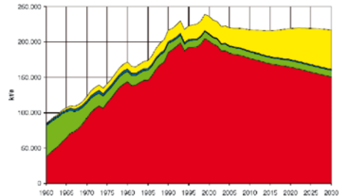
Abbildung: Kohlendioxidemissionen des Verkehrs nach Verkehrsträgern (TREMOD 2006)
